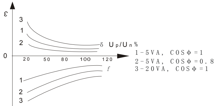
电压互感器电压与负荷特性
